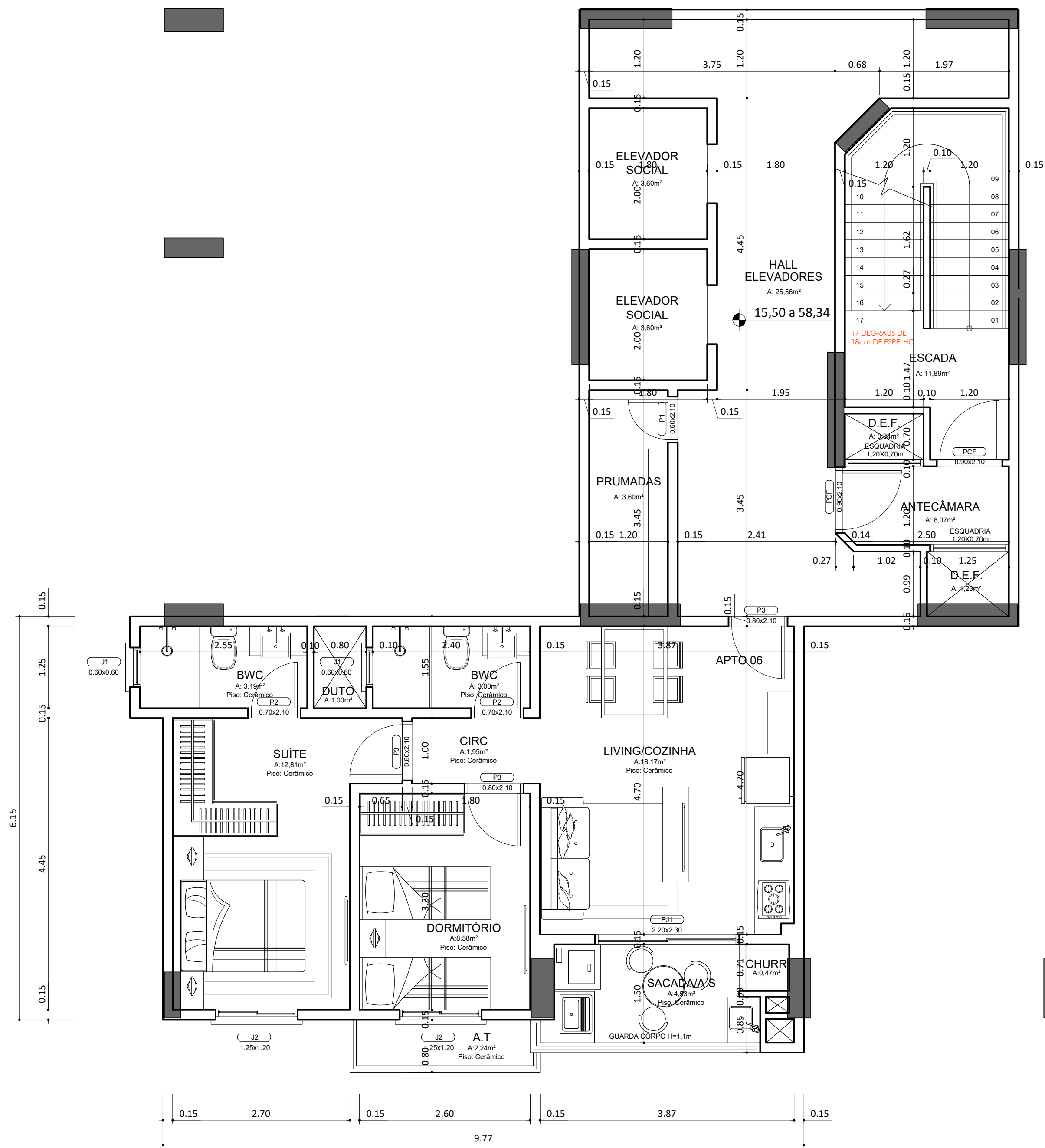
PLANTA BAIXA TIPO 06
